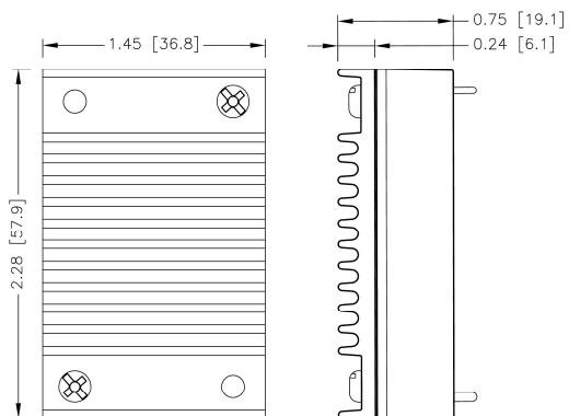
VPE40-□□S□□U – HS 7G-0029B-F
